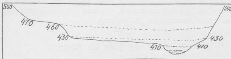
Fig. 9. Querschnitt durch das Rheintal bei Stein 1:25 000.
