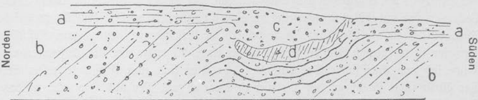
Fig. 7. Grube am Alten Bohl, nördlich von Radolfzell.
