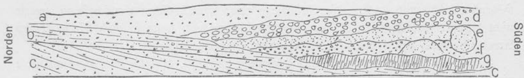
Fig. 3. Grube nördlich von Ueberlingen am Ried.
