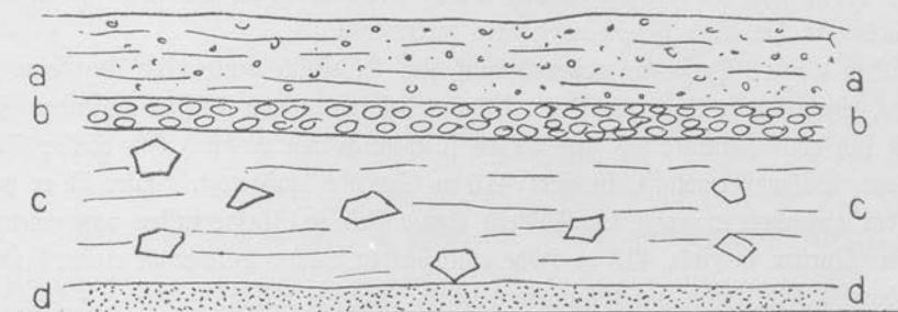
Fig. 8. Aufschluß an der Fabrik Arlen.
