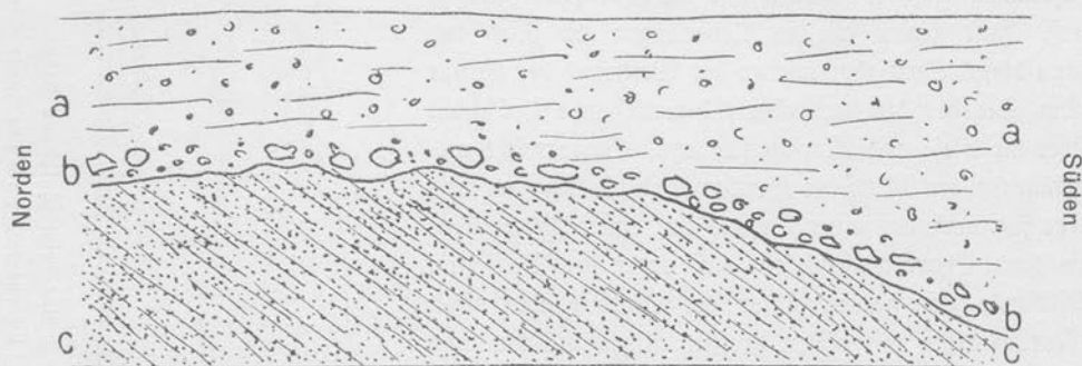
Fig. 5. Grube am Schloß Heersberg.
