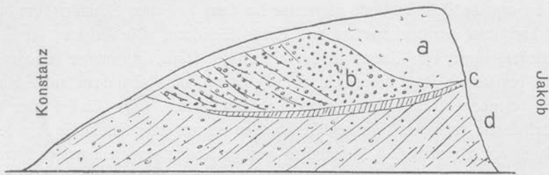
Fig. 2. Aufschluß in der Kiesgrube westlich vom Jakob bei Konstanz.
