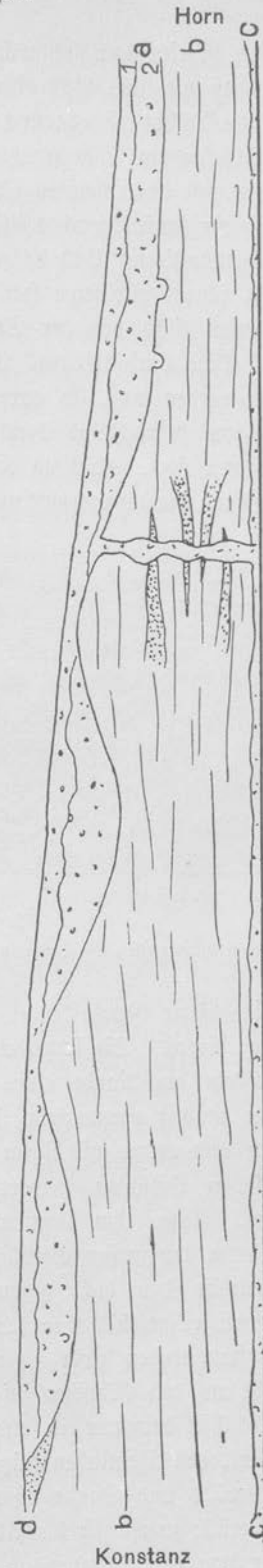
Fig. 4. Große Grube beim Waldhaus Jakob. a) Lehmmoräne, a 1 geritzt, a 2 frisch, b) horizontale Kriesschichten, c) Lehmmoräne. In b eine Spalte (Sandschichten gezeichnet) und geologische Orgeln.
