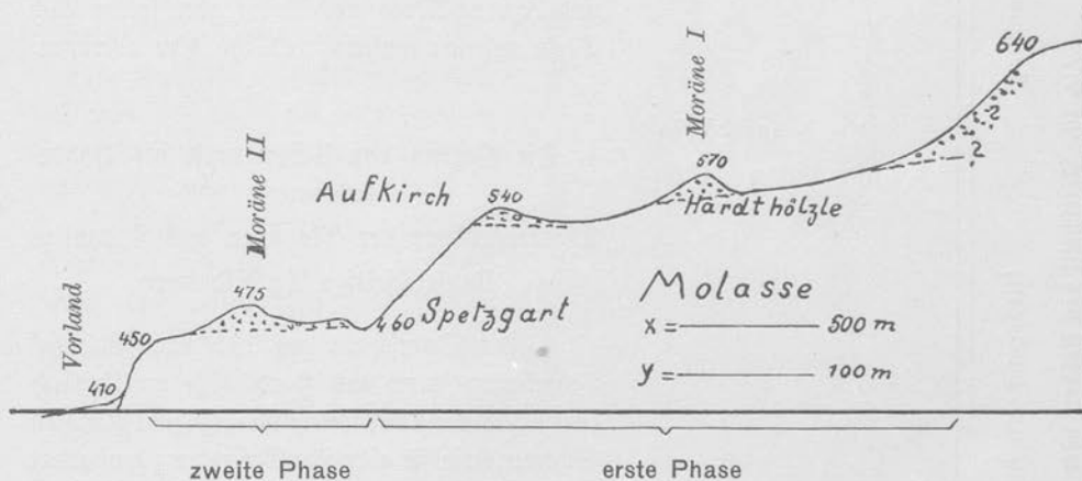
Fig. 12. Querschnitt vom Bahnhof Ueberlingen über Aufkirch.
