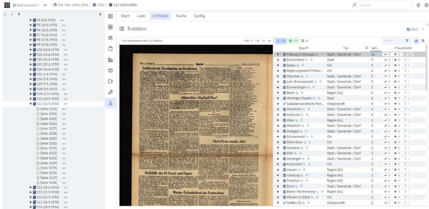
Abb. 6: Administrationsmöglichkeiten für erkannte Normdaten im VL-TextLab.
