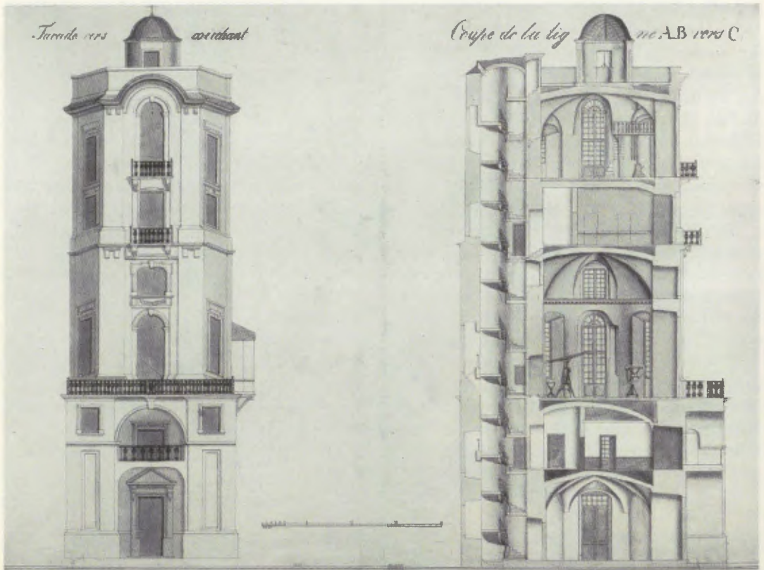
Aufriß und Querschnitt durch die Mannheimer Sternwarte. Federzeichnung, kol. von Wilhelm Traiteur, 1806, Städt. Reiss-Museum Mannheim
