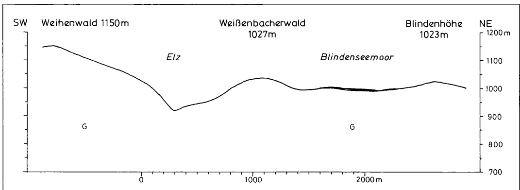
Abbildung 13. Höhenprofil des Blindenseemoors und seiner Umgebung entlang eines SW-NE-Geländeschnittes. 2,5fach überhöht. Grundlage TK 25, Bl. 7814 u. Bl. 7815. G: Granit.
