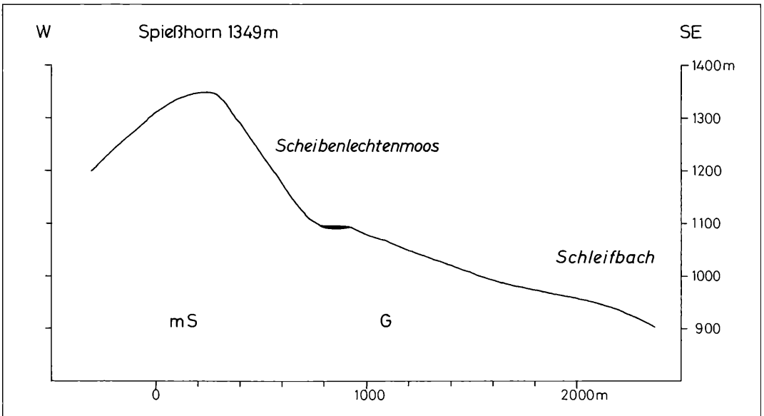
Abbildung 36. Höhenprofil des Scheibenlechtenmooses und seiner Umgebung entlang eines W-SE-Geländeschnittes. 2,5 fach überhöht. Grundlage TK 25, Bl. 8114. G: Bärhaldegranit. mS: Parametamorphite.
