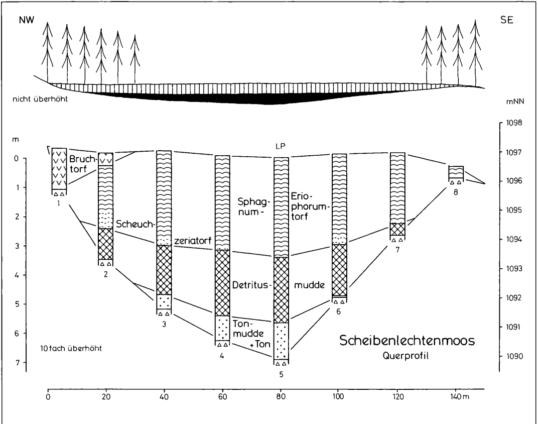
Abbildung 38. Stratigraphisches Linienprofil vom Scheibenlechtenmoos (1097 m) bei Menzenschwand (Querprofil NW-SE). Oben: Nicht überhöht, mit Vegetation. Schraffiert: Torf. Schwarz: Limnische Sedimente. Darunter: Zehnfach überhöht.
