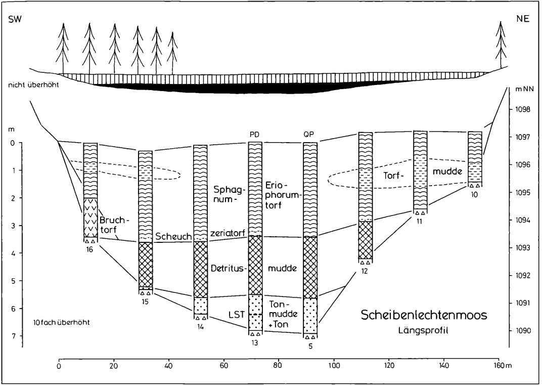
Abbildung 37. Stratigraphisches Längsprofil vom Scheibenlechtenmoos (1097 m) bei Menzenschwand (Längsprofil SW-NE). Oben: Nicht überhöht, mit Vegetation. Schraffiert: Torf. Schwarz: Limnische Sedimente. Darunter: Zehnfach überhöht.
