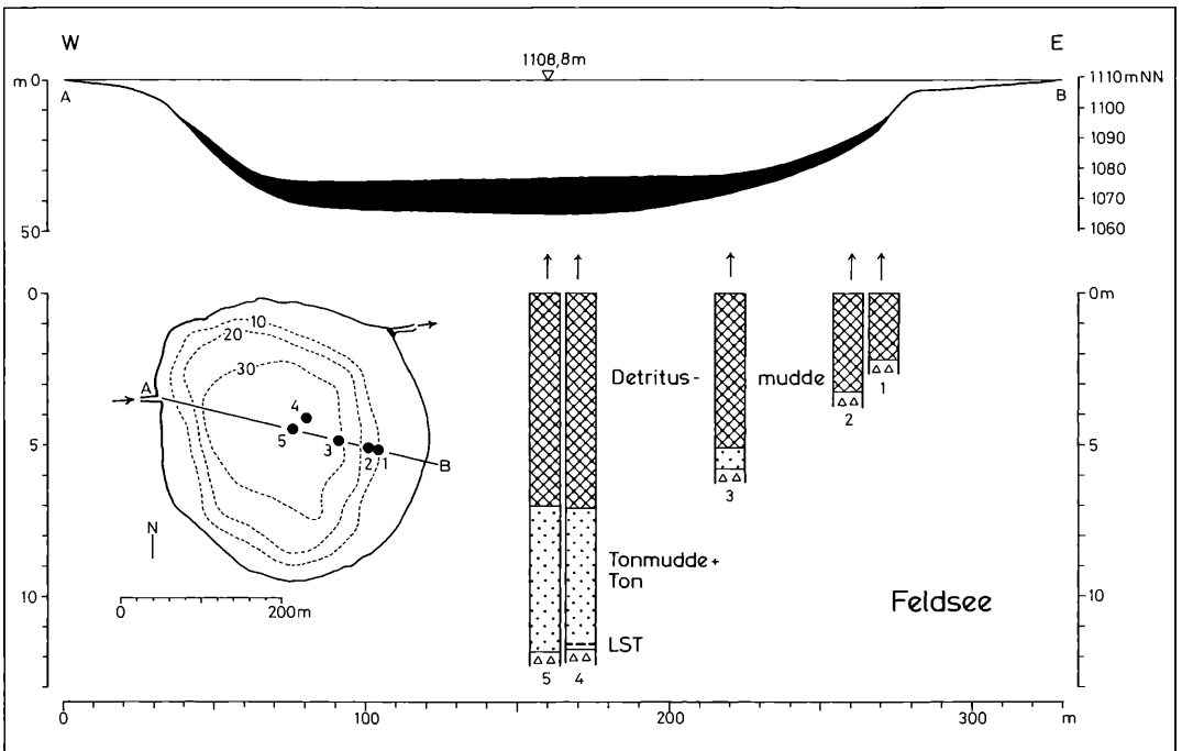
Abbildung 27. Stratigraphisches Linienprofil vom Feldsee (W-E). Oben: Nicht überhöht. Schwarz: Limnische Sedimente. Darunter: Zehnfach überhöhte Bohrprofile sowie Tiefenkarte (nach ELSTER 1961) mit Lage der Bohrpunkte.
