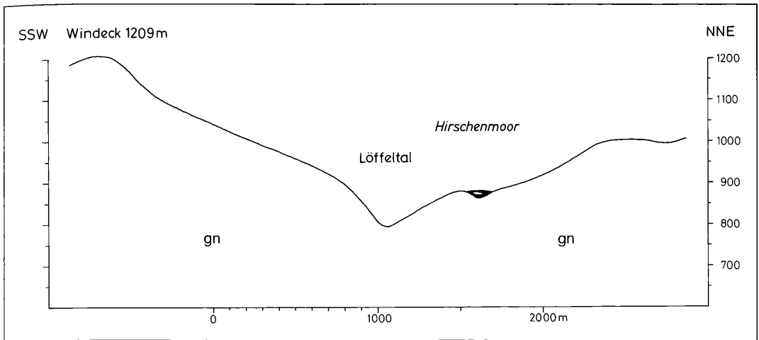
Abbildung 16. Höhenprofil des Hirschenmoores und seiner Umgebung entlang eines SSW-NNE-Geländeschnittes. 2,5 fach überhöht. Grundlage TK 25, Bl. 8014 u. Bl. 8114. gn: Gneis.
