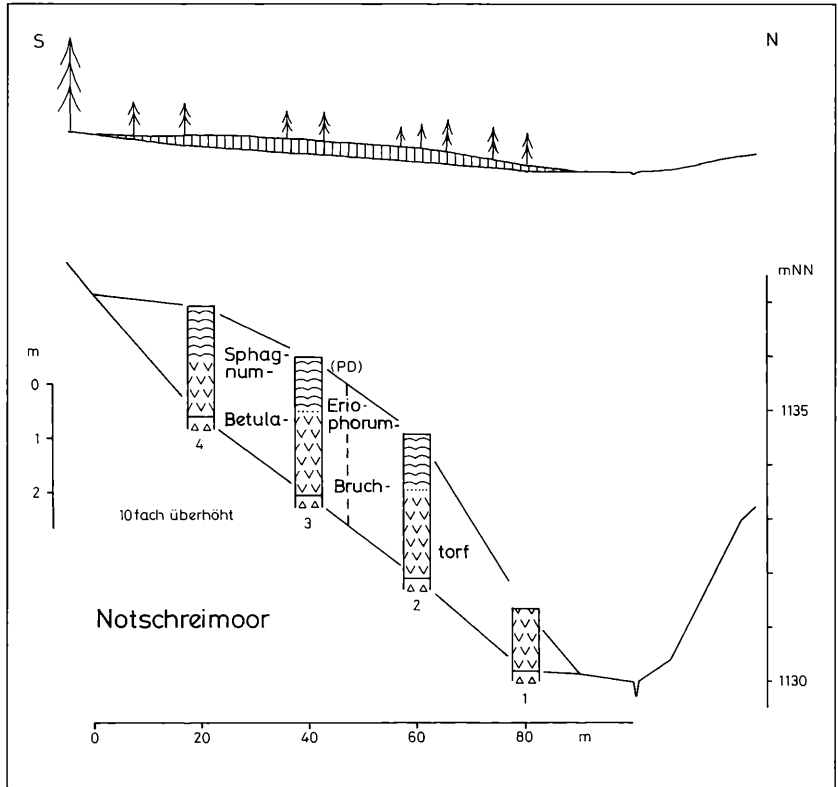
Abbildung 40. Strati- graphisches Linien- profil vom Notschrei- moor (1135 m) bei Muggenbrunn (S-N). Oben: Nicht über- höht, mit Vegetation. Schraffiert: Torf. Darunter: Zehnfach überhöht.
