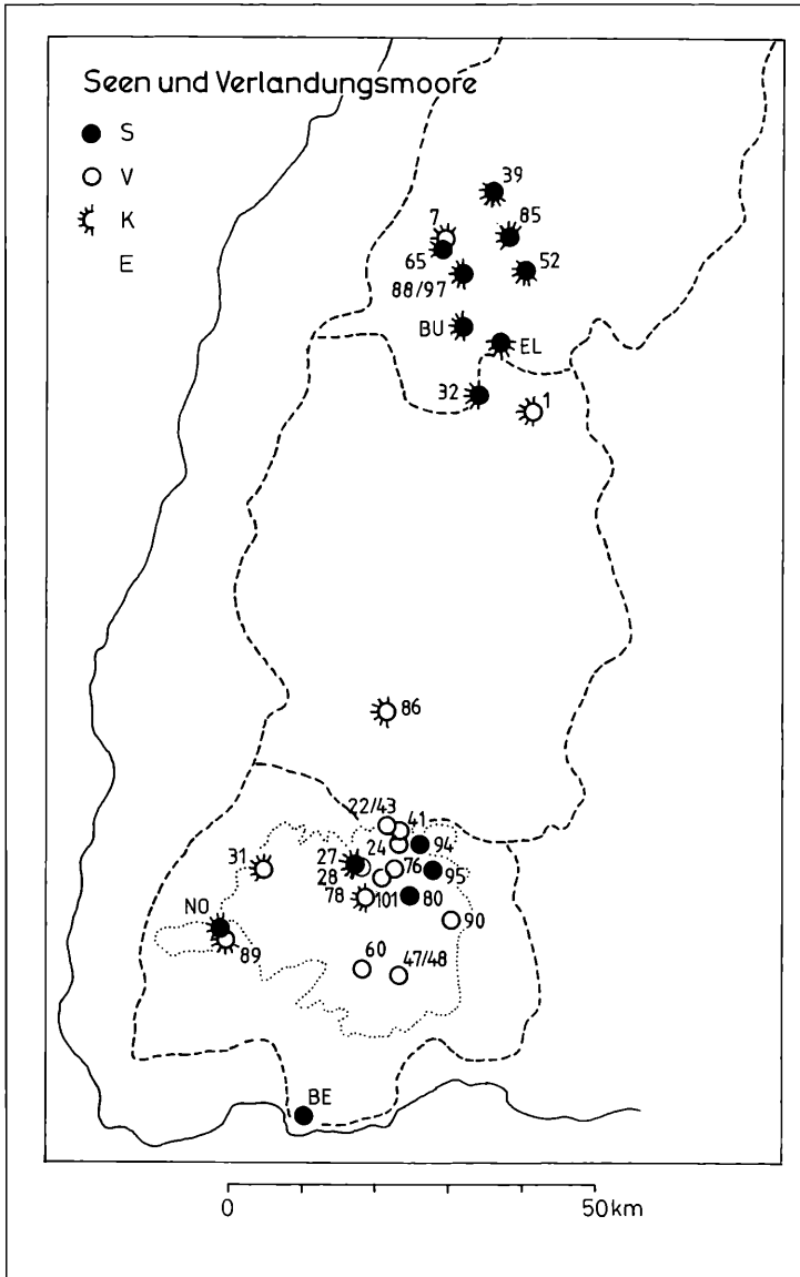
Abbildung 58. Seen und Verlandungsmoore im Schwarzwald. E: Maximale Ausdehnung der Würm-glazialen Vergletscherung im Südschwarzwald. K: Kare mit heutigen oder ehemaligen Seen. S: Heutige Seen. V: Ehemalige Seen (Verlandungsmoore). Die Ziffern beziehen sich auf die Anhangstabelle 1. BE: Bergsee (383 m). BU: Buhlbachsee (785 m). EL: Eilbchsee (770 m). NO: Nonnenmattweiher (913 m).
