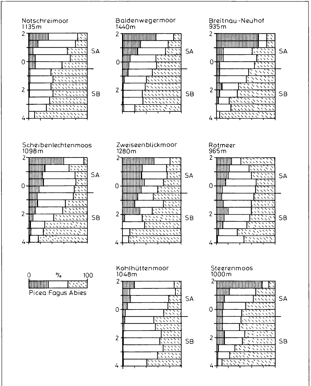
Abbildung 57. Anteile der drei Hauptholzarten Picea , Fagus und Abies im Pollenniederschlag der letzten sechstausend Jahre (Subboreal SB und Subatlantikum SA) in acht hochgelegenen Moorprofilen des Südschwarzwaldes (vgl. Abb. 56). Die Darstellung zeigt jeweils Pollen-Mittelwerte für 500 Kalenderjahre umfassende Zeitabschnitte (berechnet auf eine Pollensumme von Picea + Abies + Fagus = 100%).
