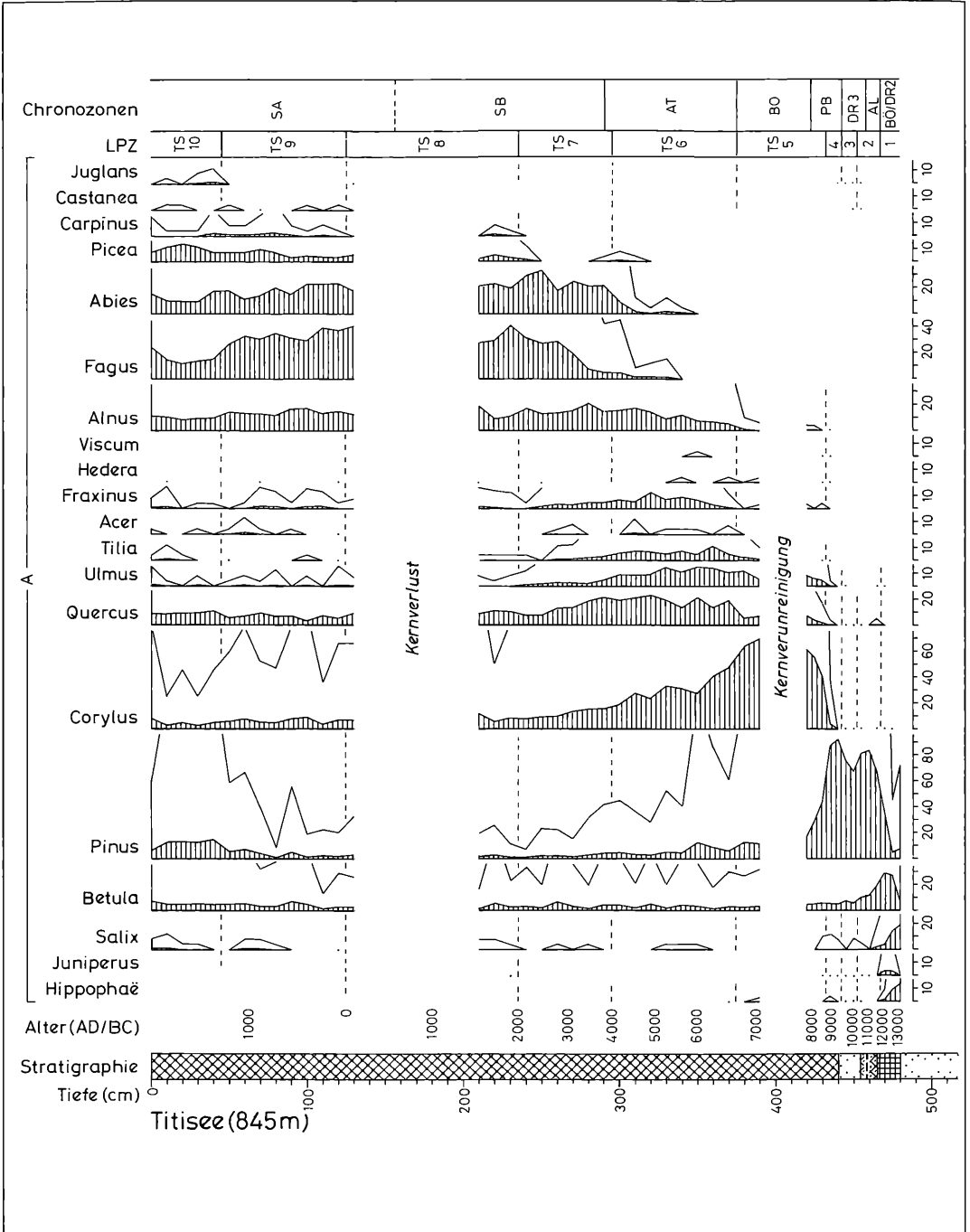
Abbildung 22a. Pollen- und Sporendiagramm vom Titisee-Nordostufer (845 m). Teil 1: Gehölzpollen. Schraffierte Silhouetten: Prozentwerte. Weiße Silhouetten: Promillewerte. Berechnungsgrundlage: Summe von Gehölzpollen (A) + Pollen terrestrischer Kräuter (B) + Pollen von Siedlungszeigern (C). Anal. G. LANG.
