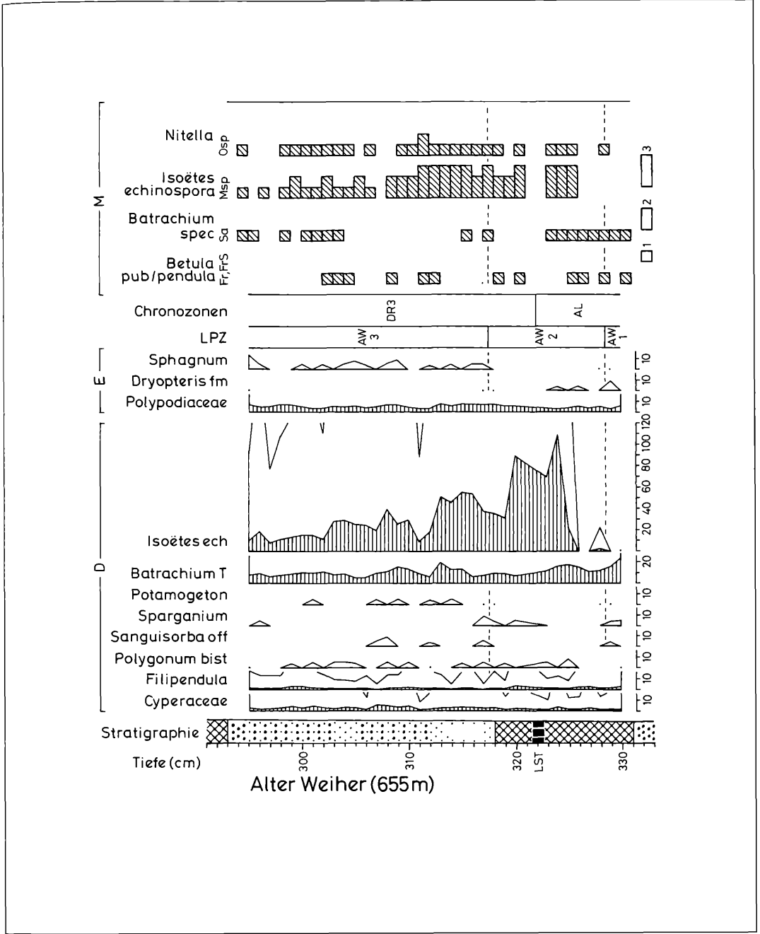
Abbildung 11b. Pollen- und Sporendiagramm sowie Großrestediagramm vom Alten Weiher (655 m) bei Freudenstadt. Spätglazialabschnitt von Bohrprofil 9. Teil 2: Pollen von Feuchtboden- und Wasserpflanzen (D), sowie Farn- und Moossporen (E). Berechnungsgrundlage: Summe von Gehölzpollen (A) + Pollen terrestrischer Kräuter (B). LST: Laacher See Tephra. Rechts daneben Großrestediagramm. Fr: Früchte, FrS: Fruchtschuppen, Msp: Megasporen, Osp: Oosporen, Sa: Samen. 1: 1-5, 2: 6-15, 3: 16 und mehr. Anal. G. LANG.
