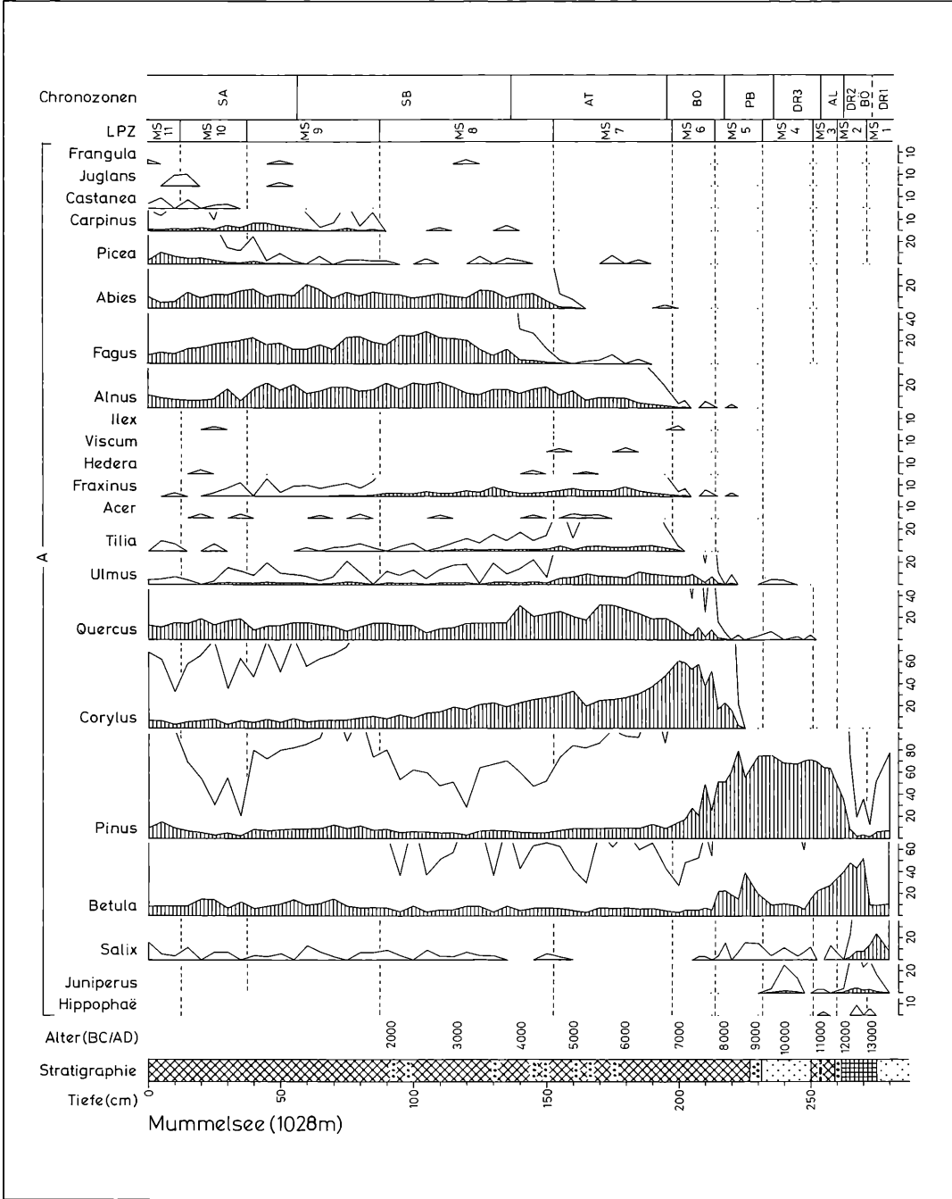
Abbildung 7a. Pollen- und Sporendiagramm vom Mummelsee (1028 m) an der Hornsgrinde. Teil 1: Gehölzpollen. Schraffierte Silhouetten: Prozentwerte. Weiße Silhouetten: Promillewerte. Berechnungsgrundlage: Summe von Gehölzpollen (A) + Pollen terrestrischer Kräuter (B) + Pollen Siedlungszeigern (C). Die Altersangaben (in kalibrierten Kalenderjahren) sind Schätzwerte auf Grund von Parallelisierungen mit 14 C-datierten Diagrammen. Anal. G. LANG.
