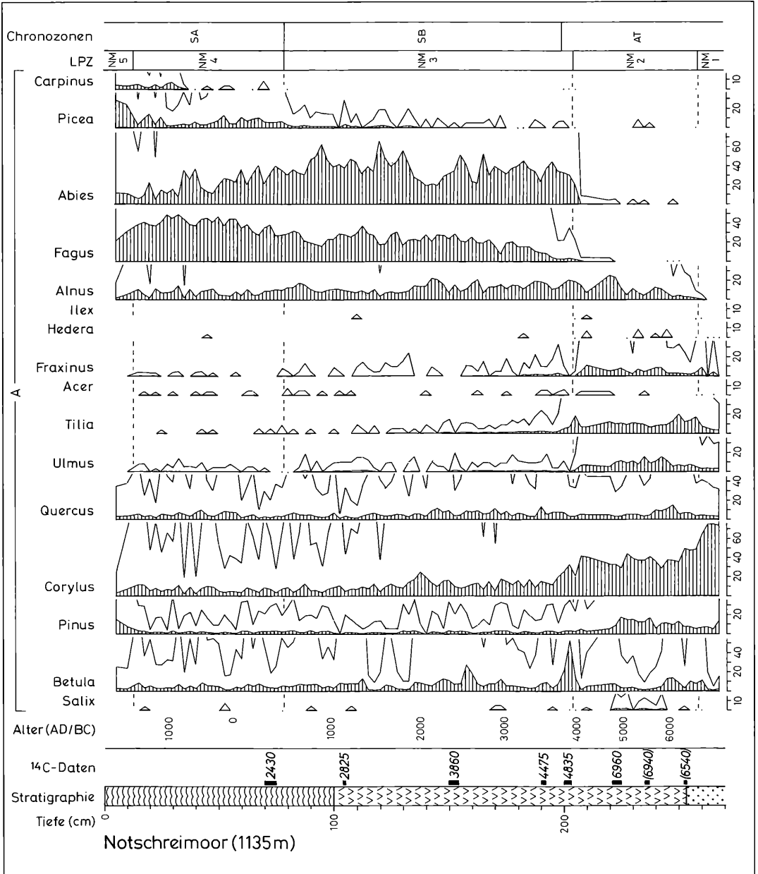
Abbildung 41a. Pollen- und Sporendiagramm vom Notschreimoor (1135 m). Teil 1: Gehölzpollen. Schraffierte Silhouetten: Prozentwerte. Weiße Silhouetten: Promillewerte. Berechnungsgrundlage: Summe von Gehölzpollen (A) + Pollen terrestrischer Kräuter (B) + Pollen von Siedlungszeigern (C). 14 C-Daten: Conv. 14 C-Jahre BP. Anal. H. WURSTER.
