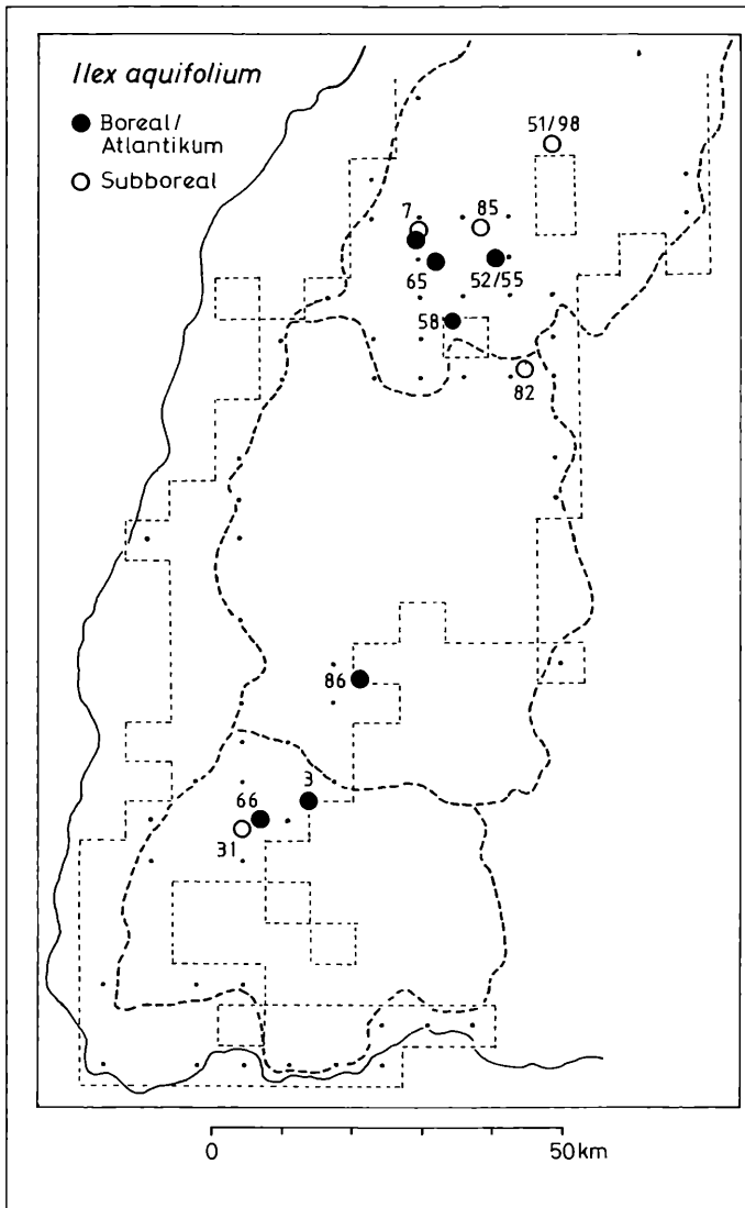
Abbildung 55. Holozäne Pollenfunde von Ilex aquifolium im Schwarzwald und heutige Verbreitung. Die Ziffern beziehen sich auf die Anhangstabelle 1. Kleine Punkte: Quadranten-Kartierung der heutigen Verbreitung im Gebiet nach SEBALD, SEYBOLD & PHILIPPI 1992.
