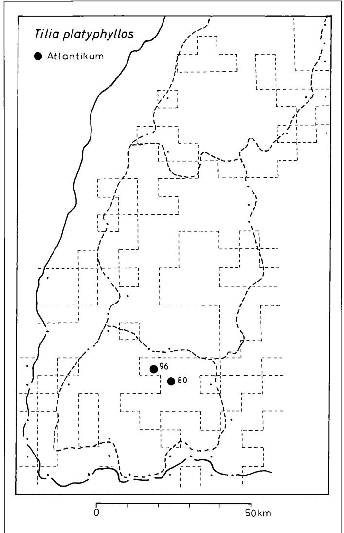
Abbildung 51. Mittelholozäne Großrestfunde von Tilia platyphyllos im Schwarzwald und heutige Verbreitung. Die Ziffern beziehen sich auf die Anhangstabelle 1. Kleine Punkte: Quadranten-Kartierung der heutigen Verbreitung im Gebiet nach SEBALD, SEYBOLD & PHILIPPI 1990b.
