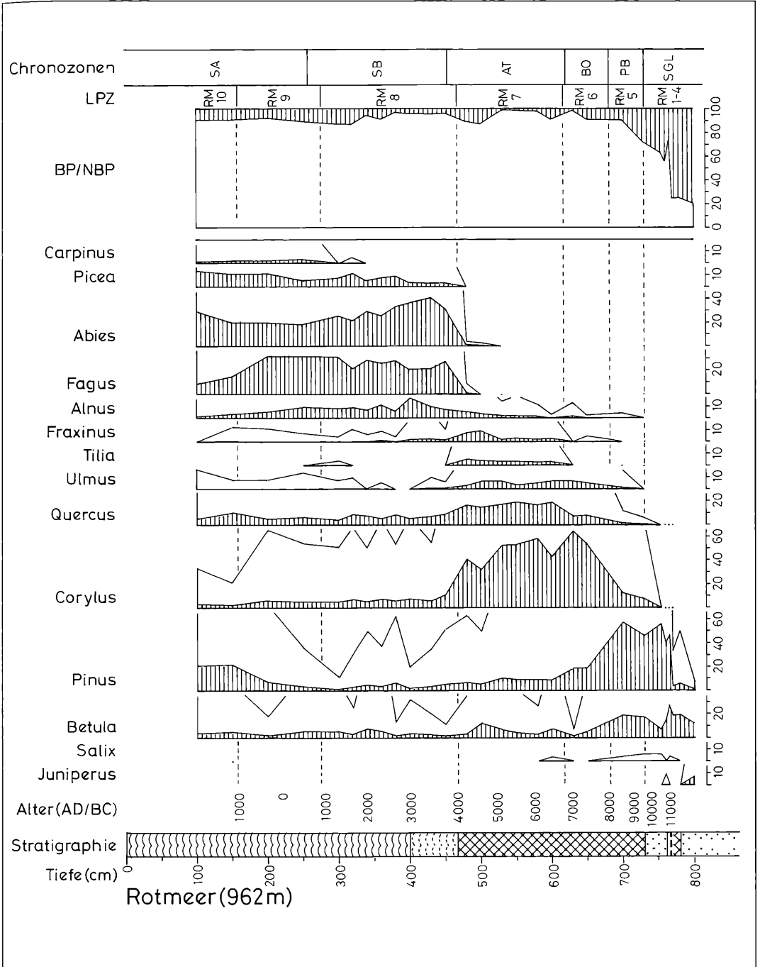
Abbildung 31. Gehölzpollendiagramm vom Rotmeer (835 m) des Profils von Bohrpunkt 6. Schraffierte Silhouetten: Prozentwerte. Weiße Silhouetten: Promillewerte. Berechnungsgrundlage: Summe der Gehölzpollen und Nicht-baumpollen (nicht differenziert). Anal. W. RAISCH.
