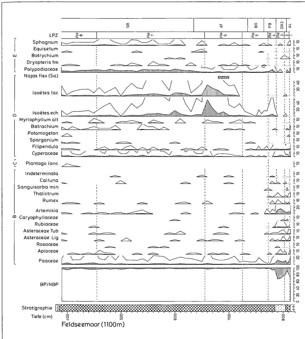
Abbildung 26b. Pollen- und Sporendiagramm vom Feldsee Moor (1100 m) von Bohrpunkt 5. Teil 2: Nichtbaumpollen und Sporen. Berechnungsgrundlage: Summe von Gehölzpollen (A) + Pollen terrestrischer Kräuter (B) + Pollen Siedlungszeigern (C). Pollen von Feuchtboden- und Wasserpflanzen (D), sowie Farn- und Moossporen (E), sind aus der Berechnungsgrundlage ausgeschlossen. Sa: Samen. Anal. G. LANG.
