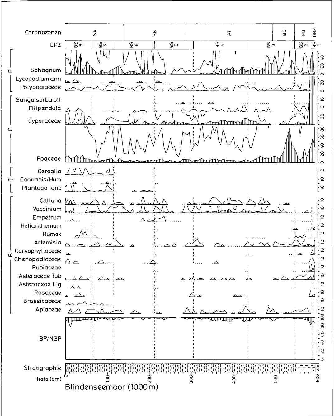
Abbildung 15b. Pollen- und Sporendiagramm vom Blindenseemoor (1000 m) bei Schonach von Bohrpunkt 8. Teil 2: Nichtbaumpollen und Sporen. Berechnungsgrundlage: Summe von Gehölzpollen (A) + Pollen terrestrischer Kräuter (B) + Pollen von Siedlungszeigern (C). Pollen von Feuchtboden- und Wasserpflanzen (D), sowie Farn- und Moossporen sind aus der Berechnungsgrundlage ausgeschlossen. Anal. C. MITTRACH.
