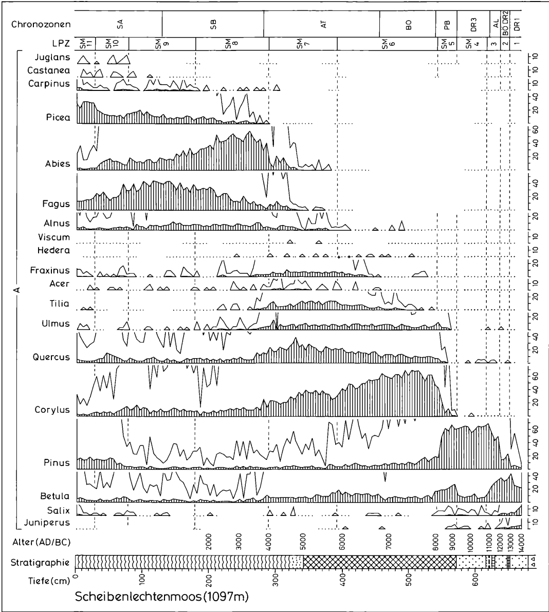
Abbildung 39a. Pollen- und Sporendiagramm vom Scheibenlechtenmoos (1097 m). Teil 1: Gehölzpollen. Schraffierte Silhouetten: Prozentwerte. Weiße Silhouetten: Promillewerte. Berechnungsgrundlage: Summe von Gehölzpollen (A) + Pollen terrestrischer Kräuter (B) + Pollen von Siedlungszeigern (C). Anal. A. SCHRÖCK (Holozän) u. G. LANG (Spätglazial).
