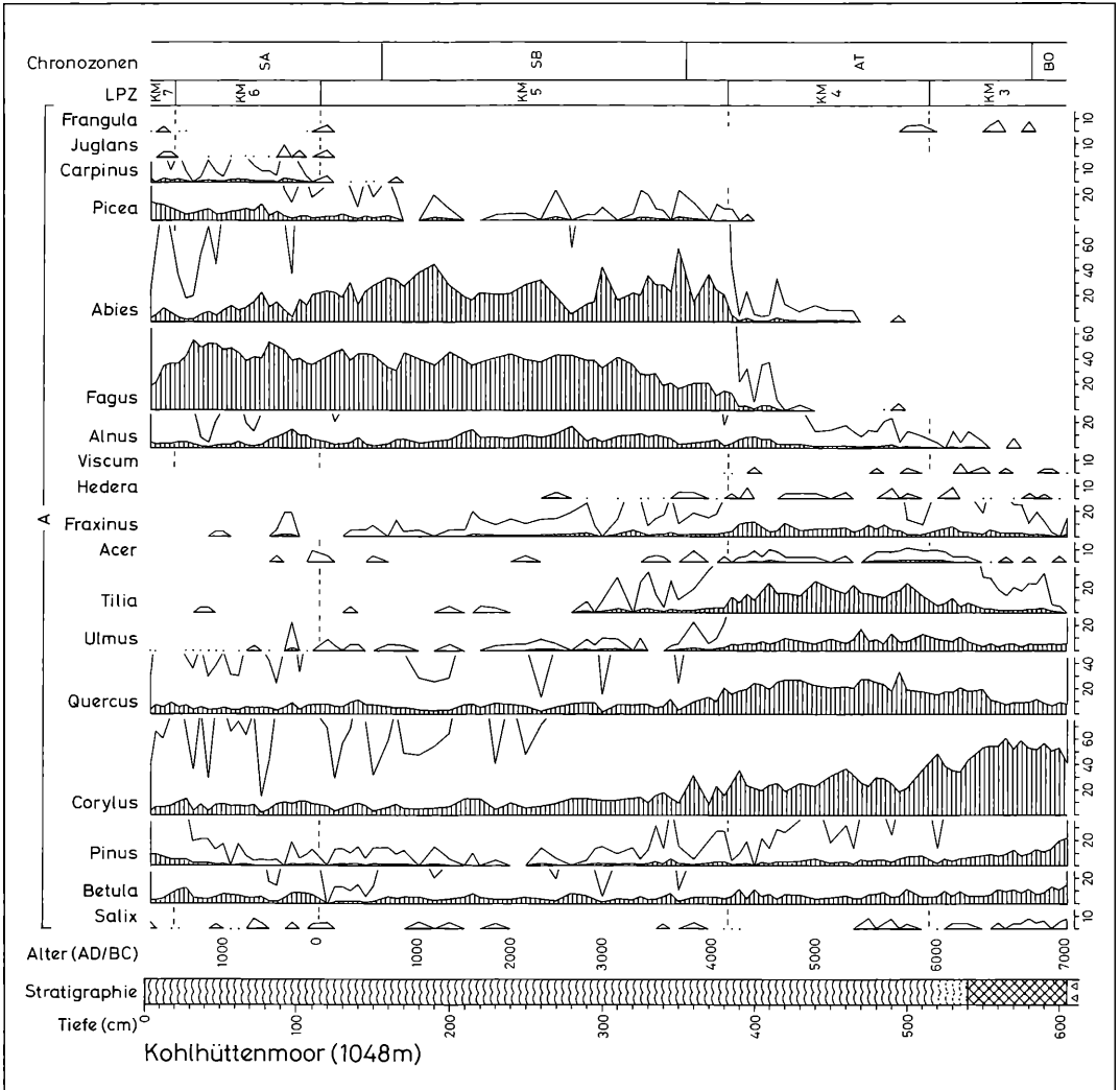
Abbildung 44a. Pollen- und Sporendiagramm vom Kohlüttenmoor (1048 m) von Bohrpunkt 15/16. Teil 1: Gehölzpollen. Schraffierte Silhouetten: Prozentwerte. Weiße Silhouetten: Promillewerte. Berechnungsgrundlage: Summe von Gehölzpollen (A) + Pollen terrestrischer Kräuter (B) + Pollen von Siedlungszeigern (C). Anal. C. SCHÄFER.
