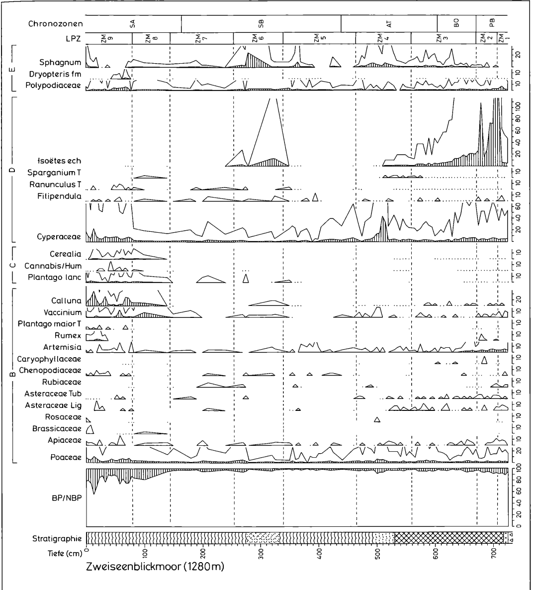
Abbildung 35b. Pollen- und Sporendiagramm vom Zweiseenblickmoor (1280 m). Teil 2: Nichtbaumpollen und Sporen. Berechnungsgrundlage: Summe von Gehölzpollen (A) + Pollen terrestrischer Kräuter (B) + Pollen von Siedlungszeigern (C). Pollen von Feuchtboden- und Wasserpflanzen (D), sowie Farn- und Moossporen (E), sind aus der Berechnungsgrundlage ausgeschlossen. Anal. U. KASTNER.
