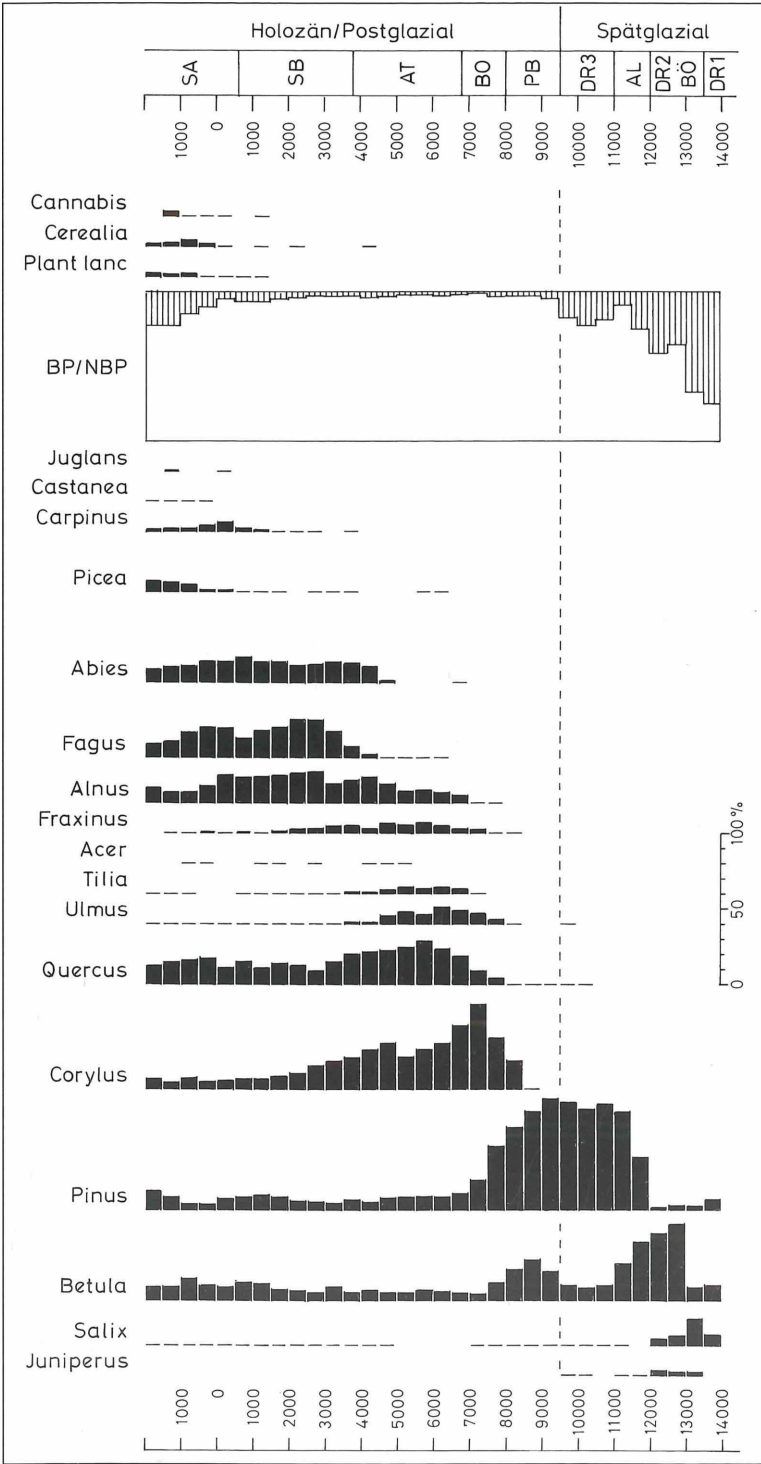
Abbildung 46. Pollendiagramm vom Mummelsee (1027 m) im Nordschwarzwald. Darstellung als Histogramm mit Mittelwerten von Gehölzpollen und Pollen einiger Siedlungszeiger für Zeitabschnitte von jeweils 500 Kalenderjahren (kalibrierte 14 C-Jahre). Vgl. dazu das Originaldiagramm (Abb. 7a u. 7b).
