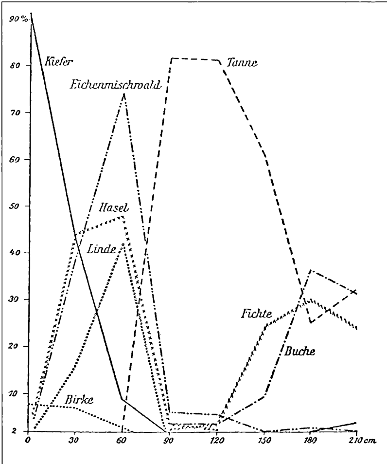
Abbildung 1. Pollendiagramm des Notschreimoors von STARK (1924). Eines der ersten Pollendiagramme aus Mitteleuropa. Im Gegensatz zur später üblichen Darstellung ist die Abszisse die Zeitachse (von links nach rechts).
