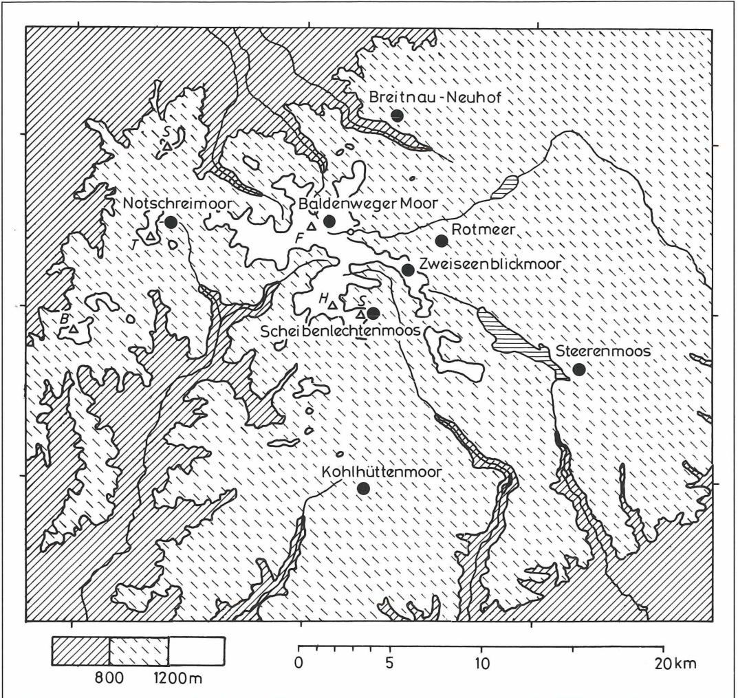
Abbildung 56. Höhenschichten-Karte des Südschwarzwalds mit Lage der untersuchten Moorprofile (Abb. 57). B: Belchen 1414 m. F: Feldberg 1493 m. H: Herzogshorn 1415 m. S: Schauinsland 1284 m/ Spießhorn 1349 m. T: Trubelsmattkopf 1281 m.
