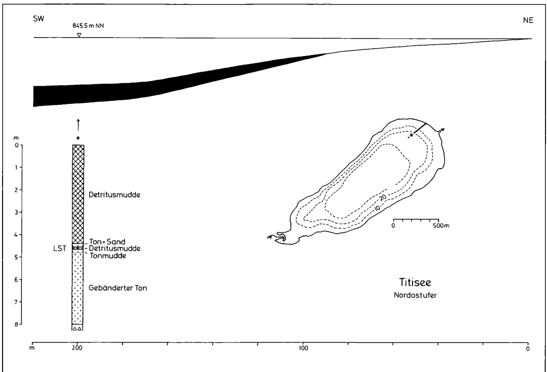
Abbildung 21. Tiefenkarte des Titisees mit Lage des Bohrprofils am Nordostufer. Oben: Nicht überhöht. Schwarz: Limnische Sedimente. Unten: Bohrprofil zehnfach überhöht. LST: Laacher See Tephra.
