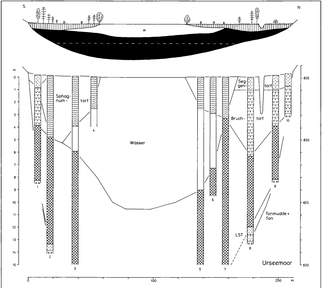
Abbildung 28. Stratigraphisches Linienprofil vom Urseemoor (835 m) bei Lenzkirch (S-N). Oben: Nicht überhöht, mit Vegetation. Schraffiert: Torf. Schwarz: Limnische Sedimente; Tiefe unterhalb der weiß gestrichelten Linie nur geschätzt. Darunter: Zehnfach überhöht.
