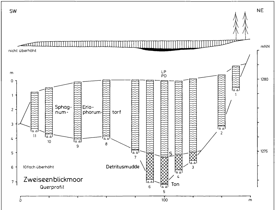
Abbildung 33. Stratigraphisches Linienprofil vom Zweiseenblickmoor (1280 m) bei Neuglashütten (Querprofil SW-NE). Oben: Nicht überhöht, mit Vegetation. Schraffiert: Torf. Schwarz: Limnische Sedimente. Darunter: Zehnfach überhöht.
