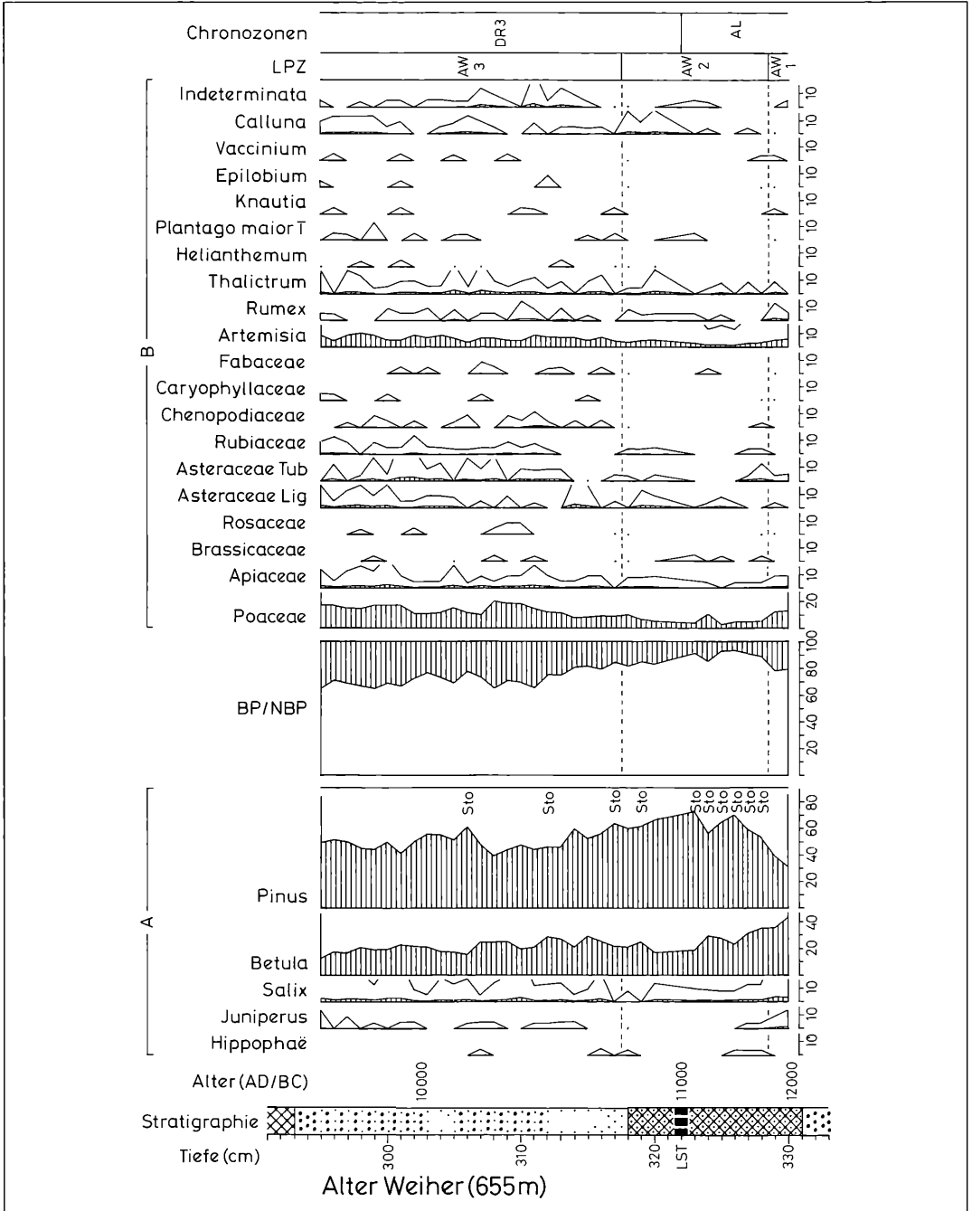
Abbildung 11a. Pollen- und Sporendiagramm vom Alten Weiher (655 m) bei Freudenstadt. Spätglazialabschnitt von Bohrprofil 9. Teil 1: Gehölzpollen und Pollen terrestrischer Kräuter. Schraffierte Silhouetten: Prozentwerte. Weiße Silhouetten: Promillewerte. Berechnungsgrundlage: Summe von Gehölzpollen (A) + Pollen terrestrischer Kräuter (B). LST: Laacher See Tephra. Sto: Pinus -Spaltöffnungen. Anal. G. LANG.
