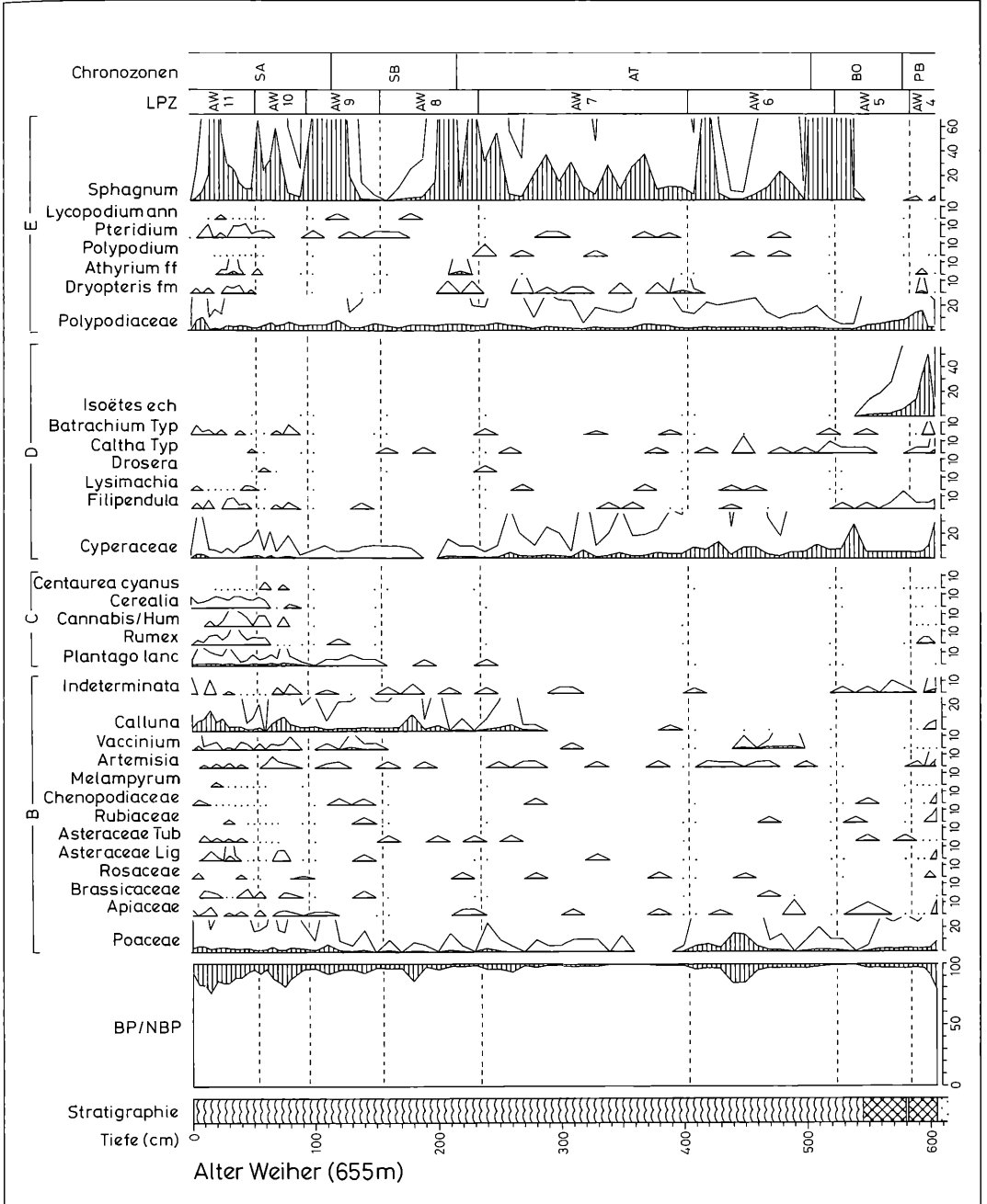
Abbildung 12b. Pollen- und Sporendiagramm vom Alten Weiher (655 m) bei Freudenstadt. Holozänabschnitt eines Profils nahe Bohrpunkt 5. Teil 2: Nichtbaumpollen und Sporen. Schraffierte Silhouetten: Prozentwerte. Weiße Silhouetten: Promillewerte. Berechnungsgrundlage: Summe von Gehölzpollen (A) + Pollen terrestrischer Kräuter (B) + Pollen von Siedungszeigern (C). Pollen von Feuchtboden- und Wasserpflanzen (D), sowie Farn- und Moosporen (E) sind aus der Berechnungsgrundlage ausgeschlossen. Anal. G. LANG.
