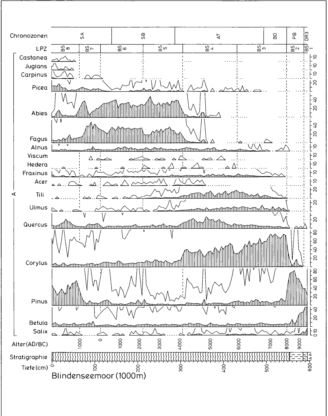
Abbildung 15a. Pollen- und Sporendiagramm vom Blindenseemoor (1000 m) bei Schonach von Bohrpunkt 8. Teil 1: Gehölzpollen. Schraffierte Silhouetten: Prozentwerte. Weiße Silhouetten: Promillewerte. Berechnungsgrundlage: Summe von Gehölzpollen (A) + Pollen terrestrischer Kräuter (B) + Pollen von Siedlungszeigern. Anal. C. MITTRACH.
