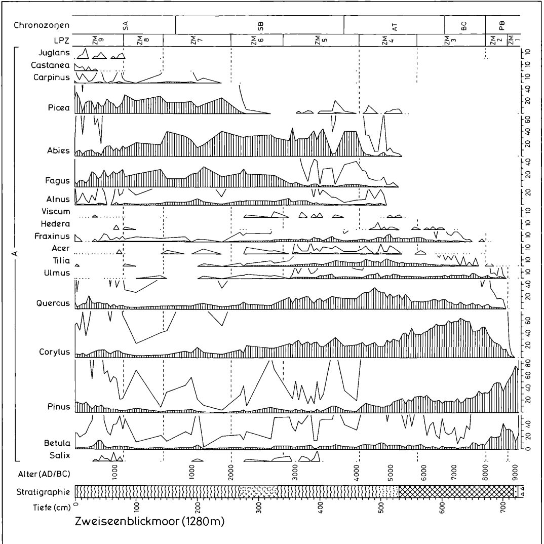
Abbildung 35a. Pollen- und Sporendiagramm vom Zweiseenblickmoor (1280 m). Teil 1: Gehölzpollen. Schraffierte Silhouetten: Prozentwerte. Weiße Silhouetten: Promillewerte. Berechnungsgrundlage: Summe von Gehölzpollen (A) + Pollen terrestrischer Kräuter (B) + Pollen von Siedlungszeigern (C). Anal. U. KASTNER.
