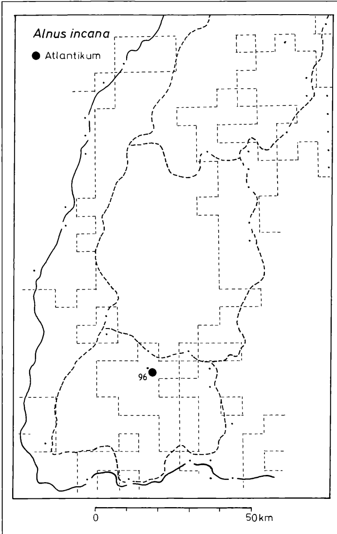
Abbildung 52. Mittelholozäner Großrestfund von Alnus incana im Schwarzwald und heutige Verbreitung. Die Ziffer bezieht sich auf die Anhangstabelle 1. Kleine Punkte: Quadranten-Kartierung der heutigen Verbreitung im Gebiet nach SEBALD, SEYBOLD & PHILIPPI 1990a.
