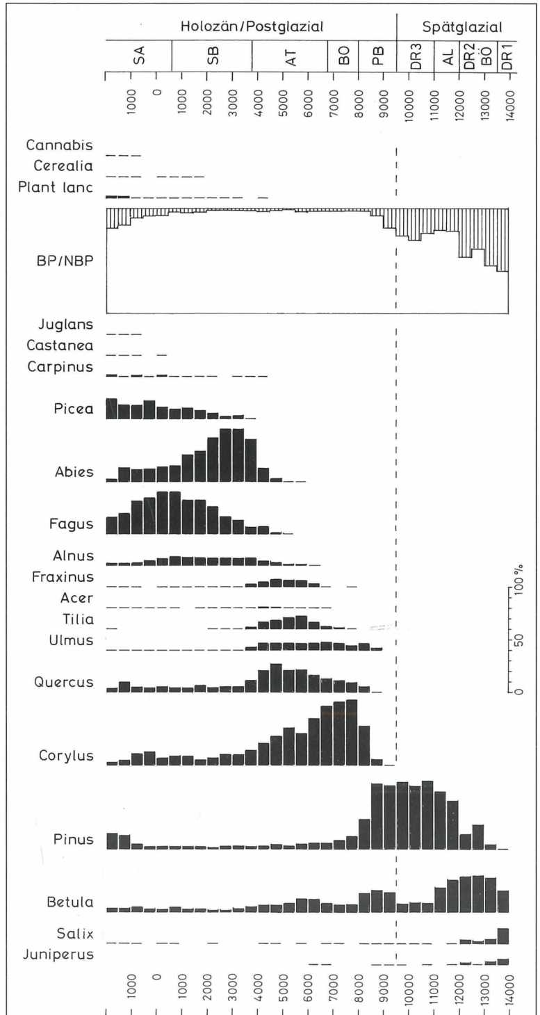
Abbildung 47. Pollendiagramm vom Scheibenlechtenmoos (1098 m) im Südschwarzwald. Darstellung als Histogramm mit Mittelwerten von Gehölzpollen und Pollen einiger Siedlungszeiger für Zeitabschnitte von jeweils 500 Kalenderjahren (kalibrierte 14 C-Jahre). Vgl. dazu das Originaldiagramm (Abb. 39a u. 39b).
