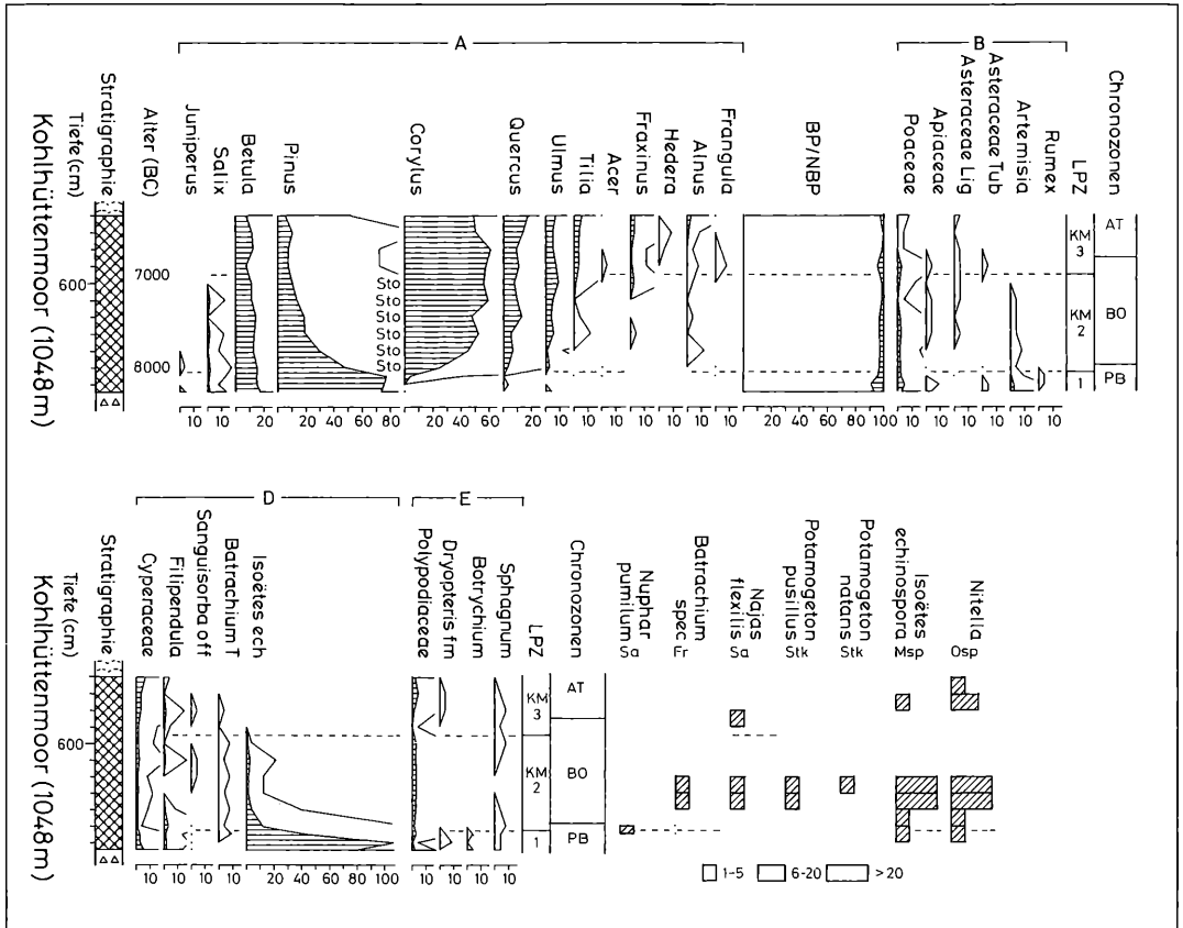
Abbildung 45. Pollen-, Sporen- und Großrestdiagramm vom Kohlhüttenmoor (1048 m) von Bohrpunkt 3 (basaler Teil). Schraffierte Silhouetten: Prozentwerte. Weiße Silhouetten: Promillewerte. Berechnungsgrundlage: Summe von Gehölzpollen (A) + Pollen terrestrischer Kräuter (B). Pollen von Feuchtboden- und Wasserpflanzen (D), sowie Farn- und Moossporen (E), sind aus der Berechnungsgrundlage ausgeschlossen. Im Großrestdiagramm bedeuten: Fr: Früchte, Msp: Megasporen, Osp: Oosporen, Sa: Samen, Stk: Steinkerne. Anal. G. LANG.
