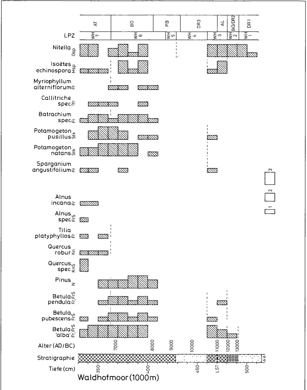
Abbildung 24c. Großrestdiagramm vom Waldhofmoor (1000 m) von Bohrpunkt 11. Fr: Früchte, FrS: Fruchtschuppen, Kn: Knospen, KnS: Knospenschuppen, Msp: Megasporen, N: Nadeln, Osp: Oosporen, Stk: Steinkerne, Tfr: Teilfrüchtchen. 1:1-5, 2:6-20; 3:>20. Anal. G. LANG.
