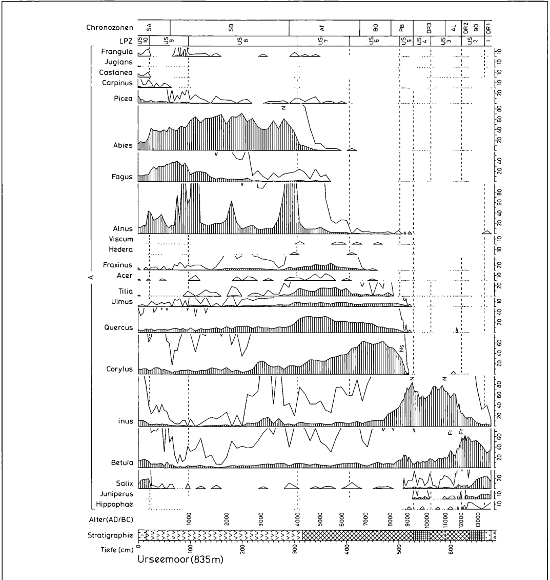
Abbildung 29a. Pollen- und Sporendiagramm vom Urseemoor (835 m). Teil 1: Gehölzpollen. Schraffierte Silhouetten: Prozentwerte. Weiße Silhouetten: Promillewerte. Berechnungsgrundlage: Summe von Gehölzpollen (A) + Pollen terrestrischer Kräuter (B) + Pollen von Siedlungszeigern (C). Anal. G. LANG.
