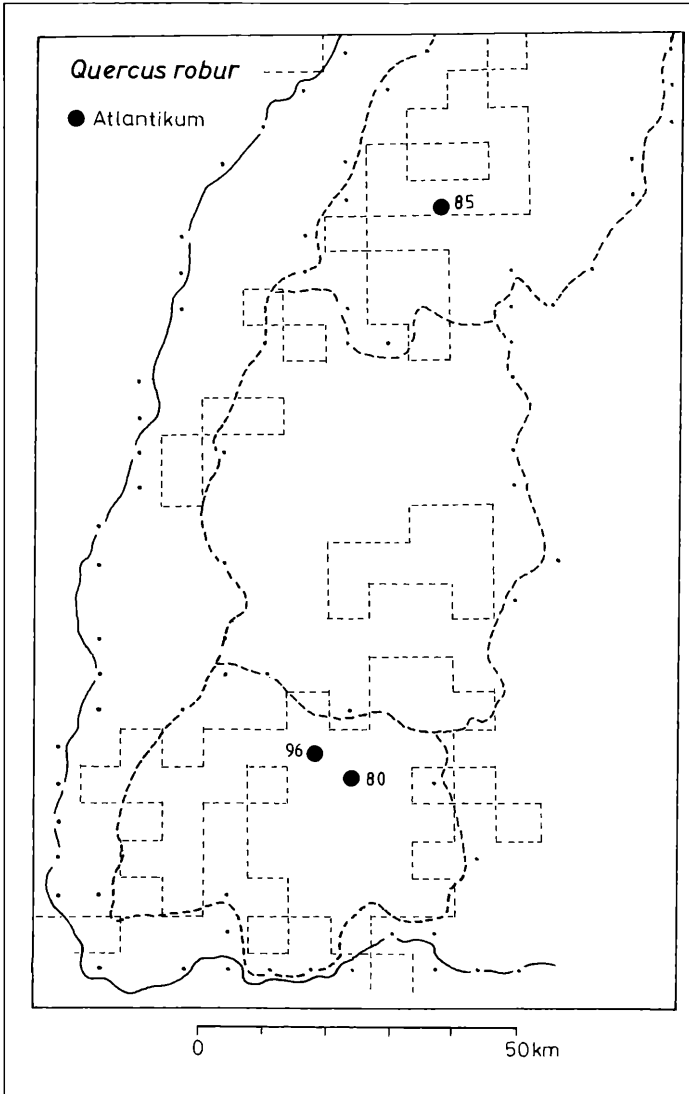
Abbildung 50. Mittelholozäne Großrestfunde von Quercus robur im Schwarzwald und heutige Verbreitung. Die Ziffern beziehen sich auf die Anhangstabelle 1. Kleine Punkte: Quadranten-Kartierung der heutigen Verbreitung im Gebiet nach SEBALD, SEYBOLD & PHILIPPI 1990a.
