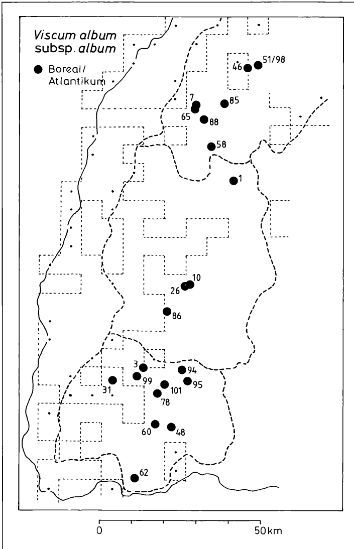
Abbildung 53. Früh- und mittelholozäne Pollenfunde von Viscum album im Schwarzwald und heutige Verbreitung. Die Ziffern beziehen sich auf die Anhangstabelle 1. Kleine Punkte: Quadranten-Kartierung der heutigen Verbreitung im Gebiet nach SEBALD, SEYBOLD & PHILIPPI 1992
