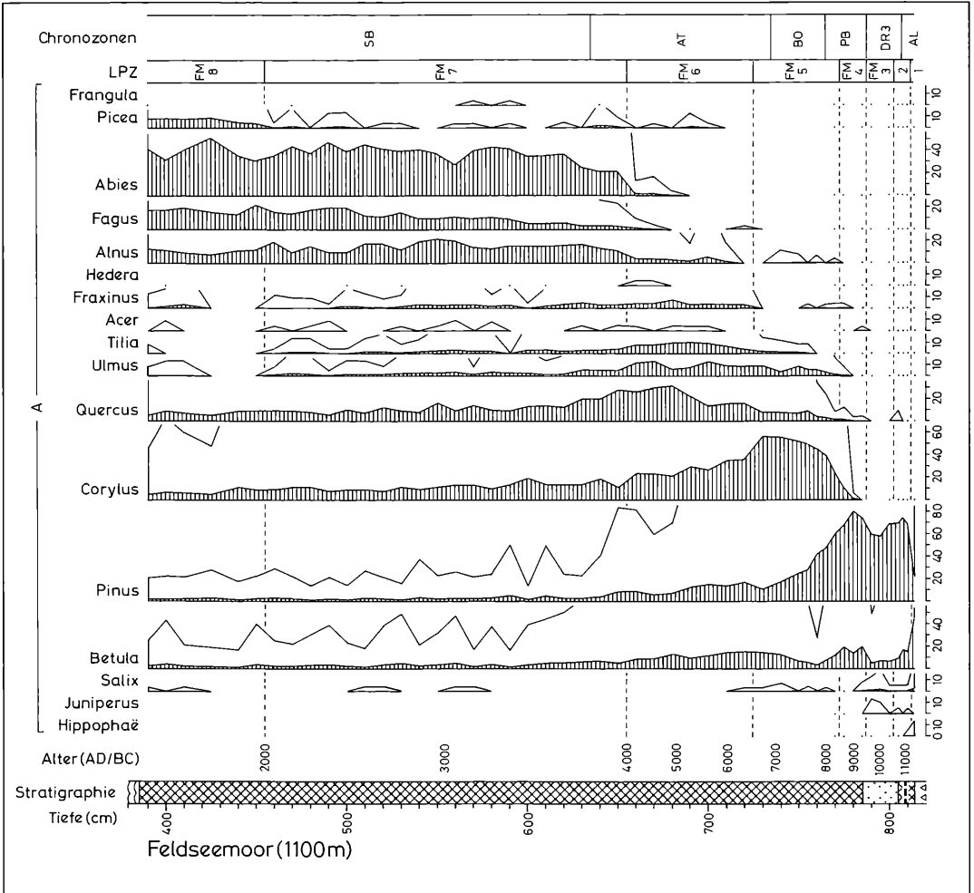
Abbildung 26a. Pollen- und Sporendiagramm vom Feldseemoor (1100 m) von Bohrpunkt 5. Teil 1: Gehölzpollen. Schraffierte Silhouetten: Prozentwerte. Weiße Silhouetten: Promillewerte. Berechnungsgrundlage: Summe von Gehölzpollen (A) + Pollen terrestrischer Kräuter (B) + Pollen von Siedlungszeigern (C). Anal. G. LANG.
