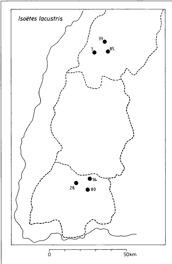
Abbildung 60. Holozäne Mikrosporenfunde von Isoëtes lacustris im Schwarzwald. Die Ziffern beziehen sich auf die Anhangstabelle 1.
