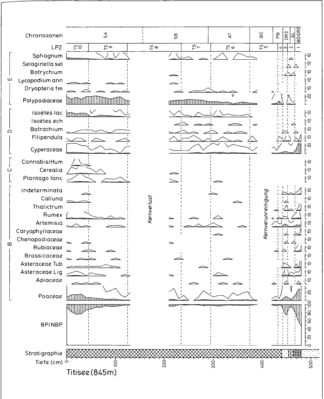
Abbildung 22b. Pollen- und Sporendiagramm vom Titisee-Nordostufer (845 m). Teil 2: Nichtbaumpollen und Sporen. Schraffierte Silhouetten: Prozentwerte. Weiße Silhouetten: Promillewerte. Berechnungsgrundlage: Summe von Gehölzpollen (A) + Pollen terrestrischer Kräuter (B) + Pollen von Siedlungszeigern (C). Pollen von Feuchtboden- und Wasserpflanzen (D) sowie Farn- und Moossporen (E) sind aus der Berechnungsgrundlage ausgeschlossen. Anal. G. LANG.
