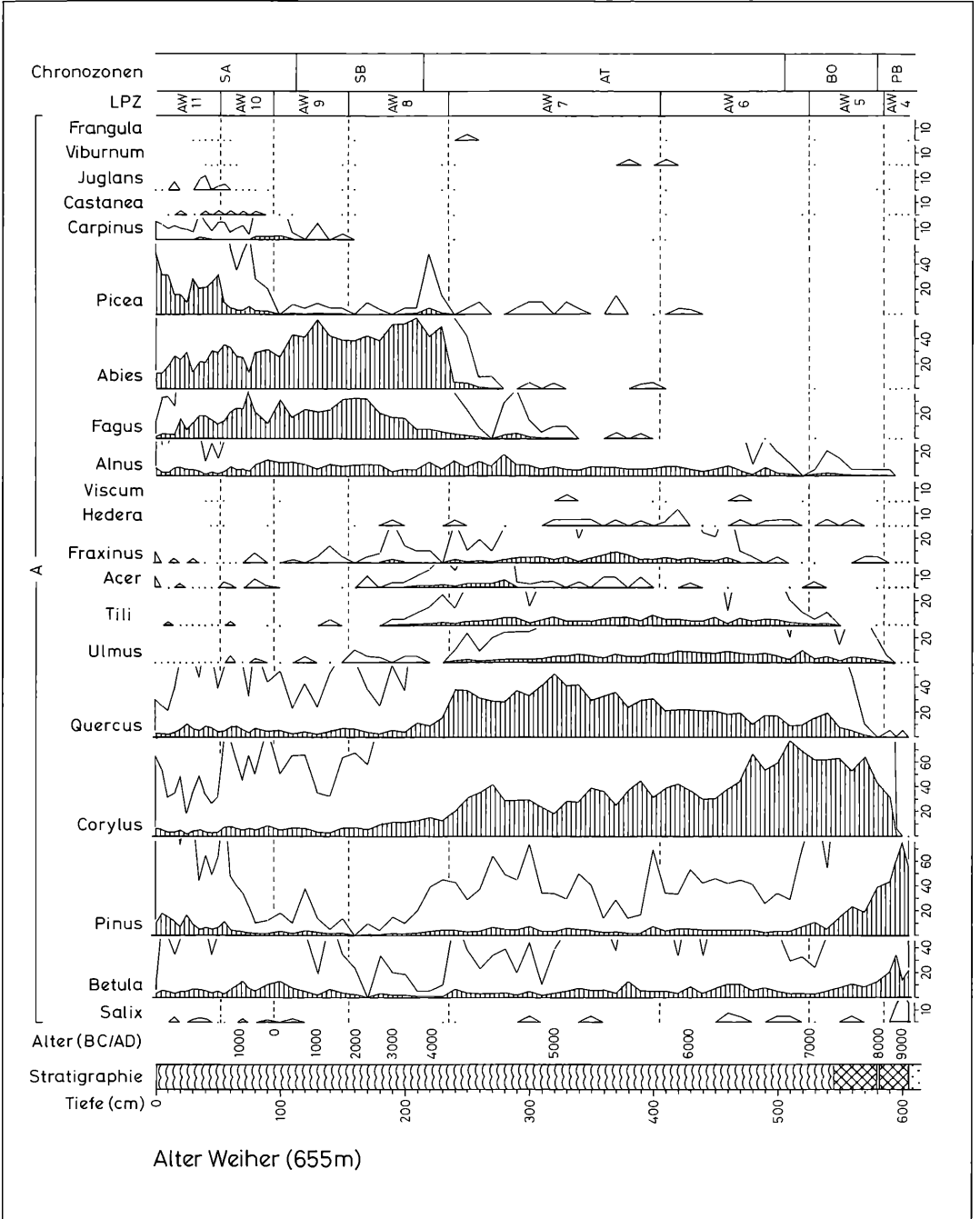
Abbildung 12a. Pollen- und Sporendiagramm vom Alten Weiher (655 m) bei Freudenstadt. Holozänabschnitt eines Profils nahe Bohrpunkt 5. Teil 1: Gehölzpollen. Schraffierte Silhouetten: Prozentwerte. Weiße Silhouetten: Promillewerte. Berechnungsgrundlage: Summe von Gehölzpollen (A) + Pollen terrestrischer Kräuter (B) + Pollen von Siedlungszeigern (C). Anal. G. LANG.
