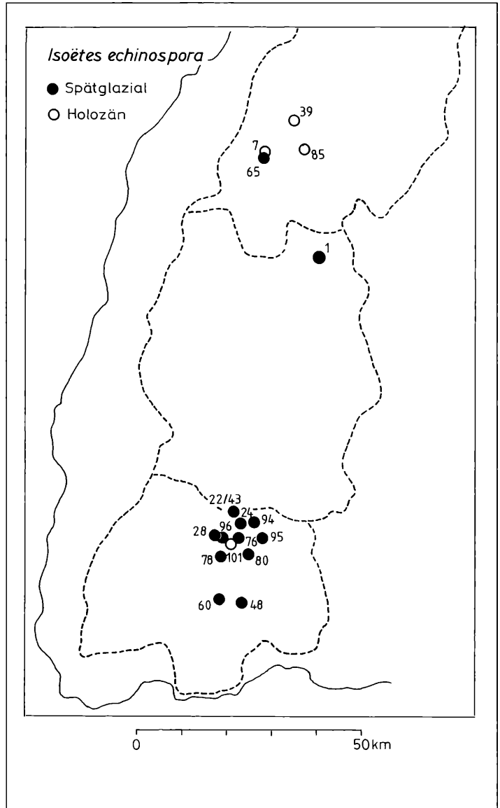
Abbildung 59. Spätglaziale und holozäne Sporenfunde (Mikro- und Megasporen) von Isoëtes echinospora im Schwarzwald. Die Ziffern beziehen sich auf die Anhangstabelle 1.
