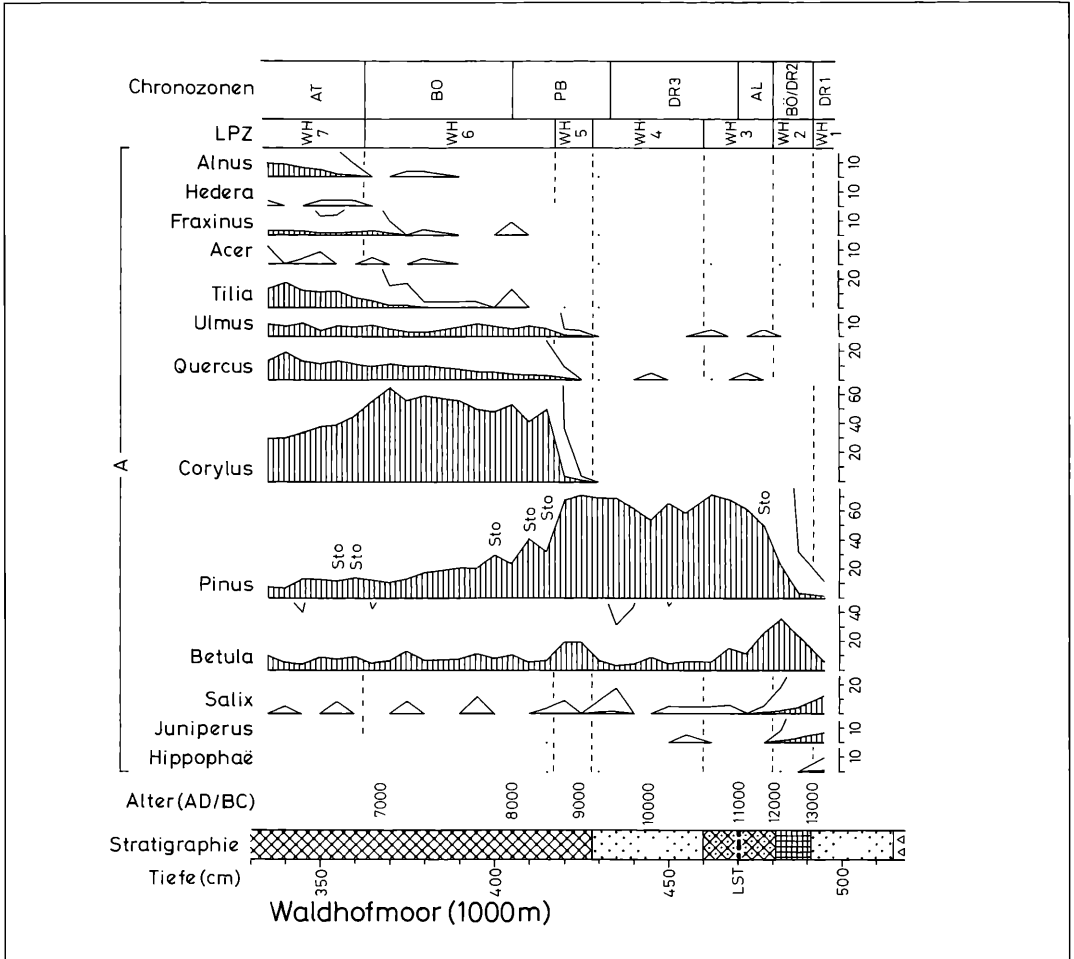
Abbildung 24a. Pollen- und Sporendiagramm vom Waldhofmoor (1000 m) von Bohrpunkt 11. Teil 1: Gehölzpollen. Schraffierte Silhouetten: Prozentwerte. Weiße Silhouetten: Promillewerte. Berechnungsgrundlage: Summe von Gehölzpollen (A) + Pollen terrestrischer Kräuter (B). Anal. G. LANG.
