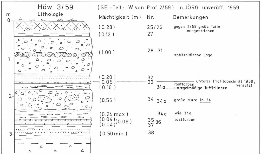
Abbildung 9. Profil Höw 3/59 der Höwenegg-Schichten im SE-Teil der Grabungsstelle 1, W von Höw 2/59 (nach JÖRG 1959, unveröff.; Kap. 6.1, Grabungsstellen). Obermiozän, Höwenegg, Südwestdeutschland.
