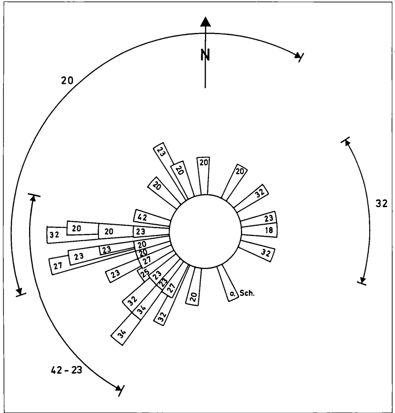
Abbildung 28. Einstreuung der Säugetierskelette der Höwenegg-Schichten in allen Fundschichten der Grabungsstelle 1 mit Angabe der Kopforientierung. Jedes Feld bedeutet ein Individuum (n=31), nicht unterteilte lange Felder (Bsp. 27 nach WSW) ergeben sich aber aus der Darstellung. Die beiden Kreissegmente geben für bestimmte Schichten hervortretende Richtungen an. Obermiozän, Höwenegg, Südwestdeutschland.
