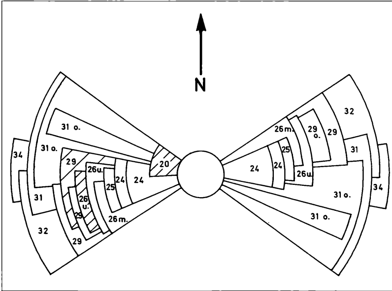
Abbildung 27 Übereinanderprojektion der Hauptsektoren der Einstuerungsmessungen an der Grabungsstelle 1 in den einzelnen Schichten der Höwenegg-Schichten. Polare Elemente sind durch Schraffur gekennzeichnet. Die Länge der Sektorendarstellung ist ohne Bedeutung, sie ergibt sich aus der Übereinanderprojektion. Obermiozän, Höwenegg, Südwestdeutschland.
