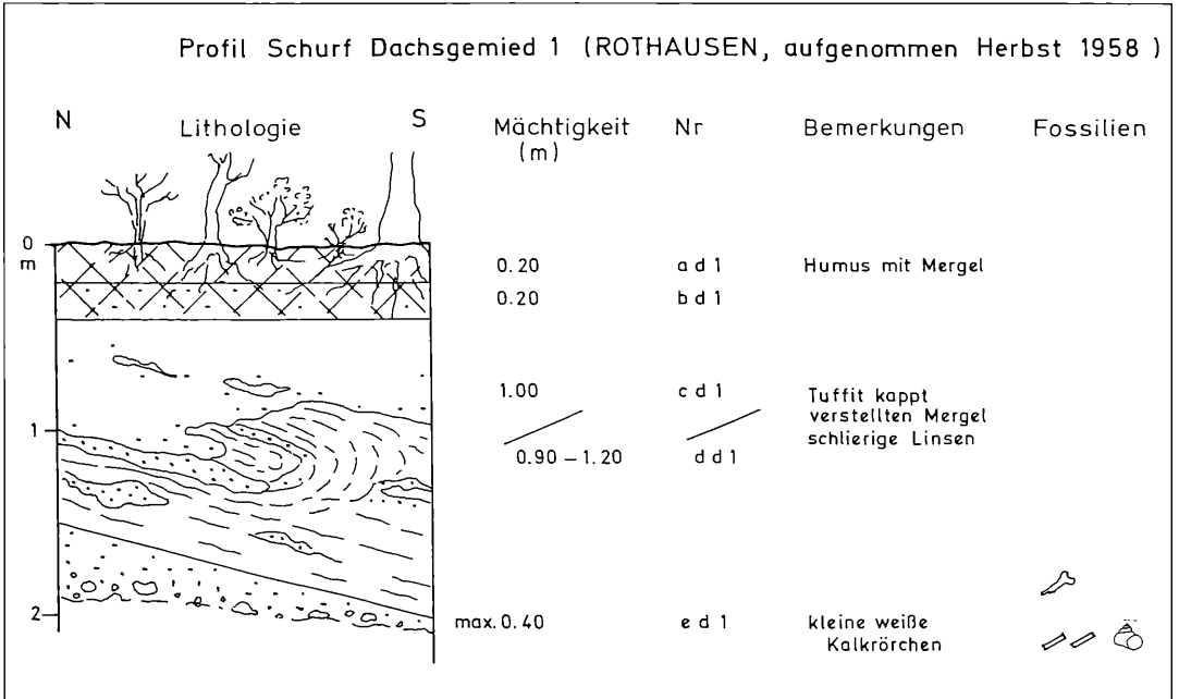
Abbildung 20. Profil Schurf Dachsgemied 1 der Höwenegg-Schichten, etwa 875 m E der Grabungsstelle 1 (nach ROTHHAUSEN 1958, unveröff.; Kap. 6.1.2, Schürfe). Obermiozän, Höwenegg, Südwestdeutschland.
