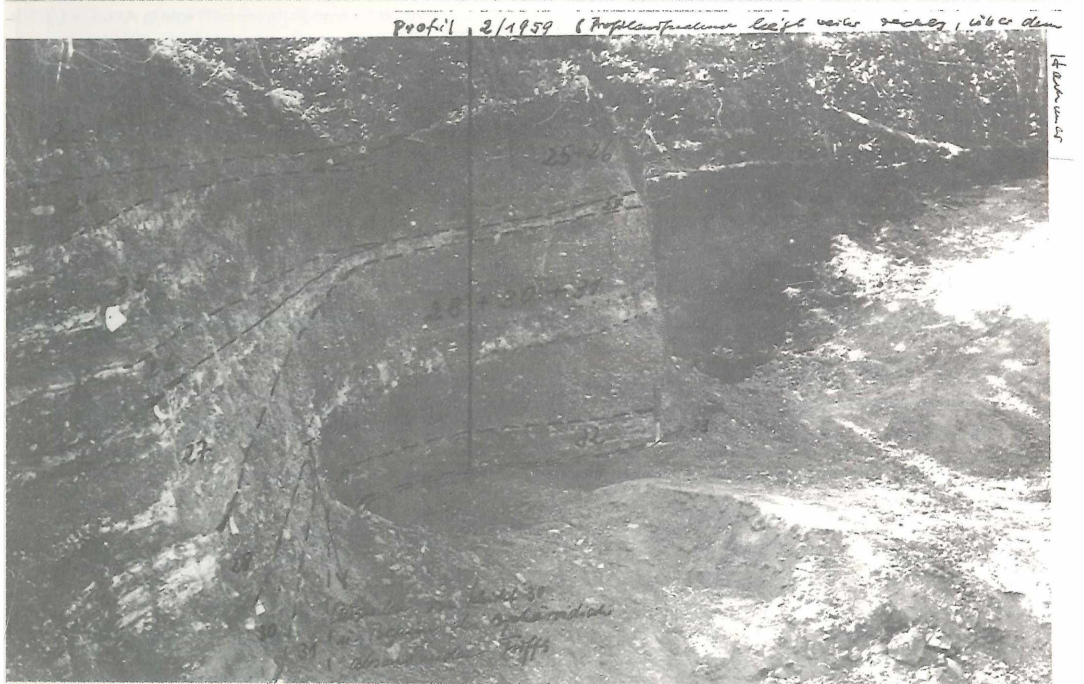
Abbildung 6a. Profil der Höweneggschichten im SE-Teil der Grabungsstelle (Foto mit Eintragung von JÖRG 1959), entsprechend Höw 2/59 (Abbildung 7). Obermiozän, Höwenegg, Südwestdeutschland.- Aufnahme von NW. Abbildung 6b. Wie Aufnahme Abb.6a von NE.
