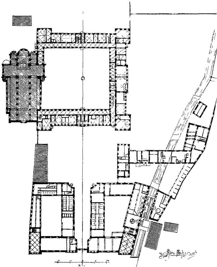
Abb. 2. Grundriß.
