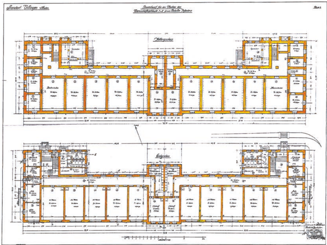
Abb. 6: Villingen. Mannschaftsgebäude. Grundriss (Stadt Villingen-Schwenningen, Bauaktenarchiv, ID Nr. 515 117.3)
